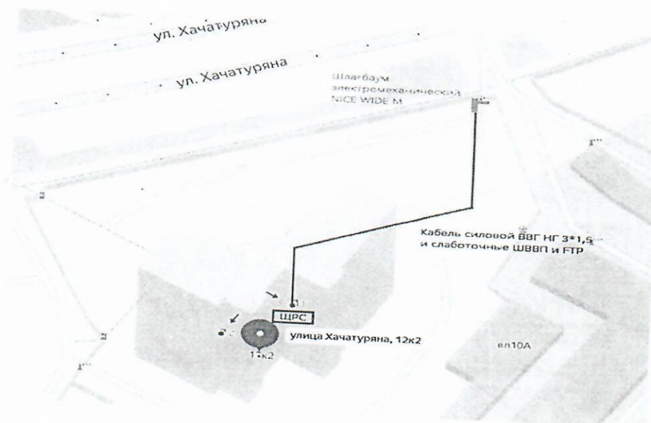
Рис. 1 Схема размещения шлагбаумов
